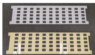
開発した25%開口率の塞ぎ板2枚を重ねて使用します。
